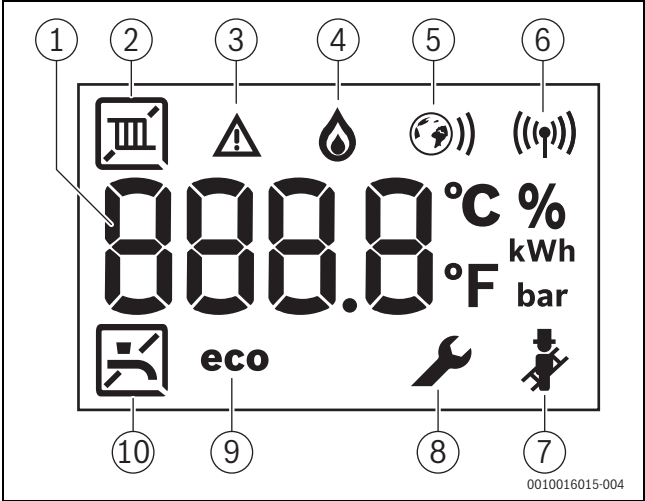
Fig. 7 Screen display
