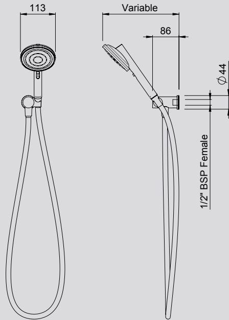
TŪROA HAND SHOWER
