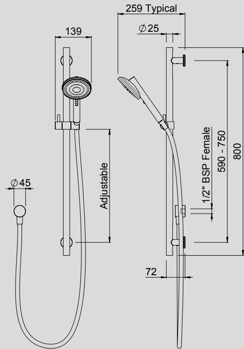
TŪROA RAIL SHOWER
