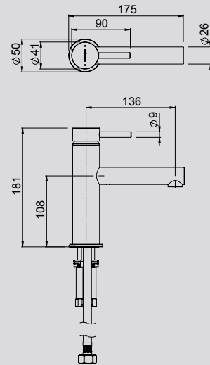
TŪROA BASIN MIXER
